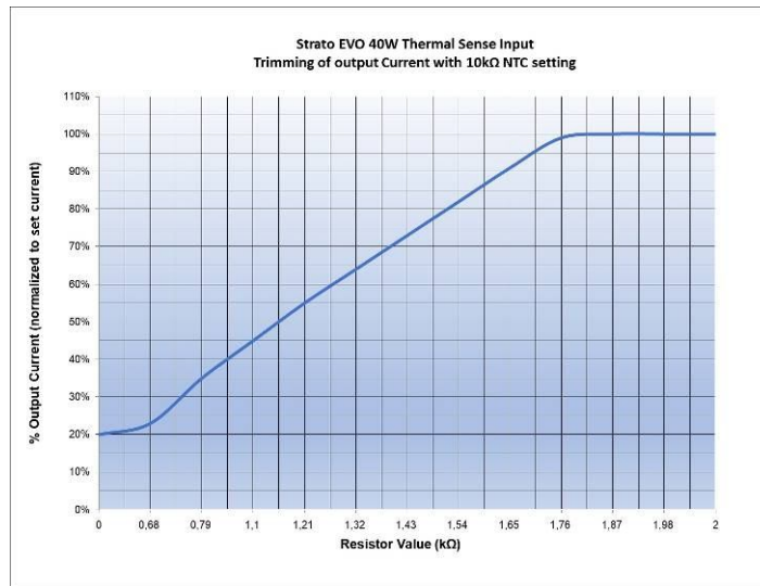
10 KΩ NTC
