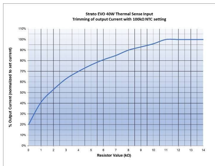
100 KΩ NTC
